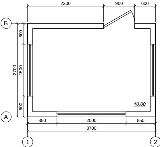
План ( 10 м²)
