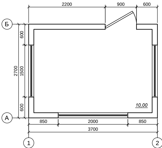
План ( 10 м²)
