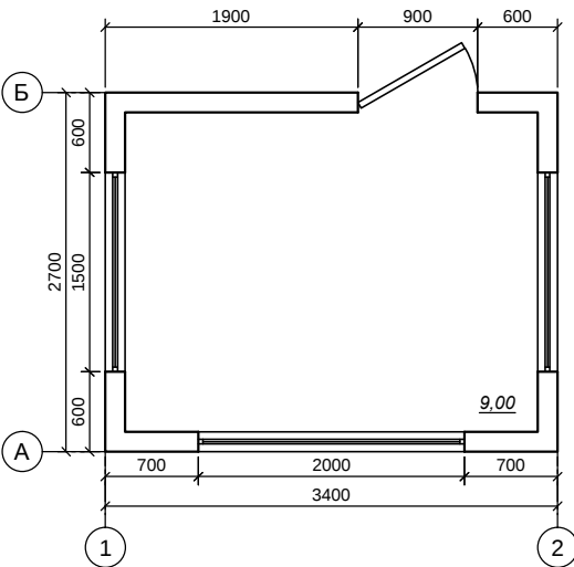
План ( 9 м²)
