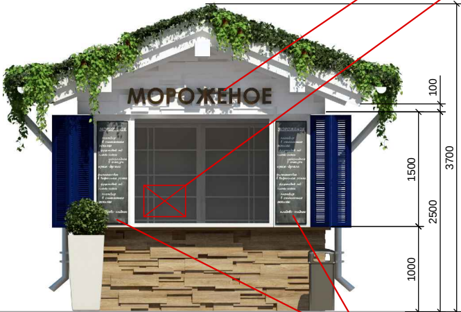
Фасад 1-2
