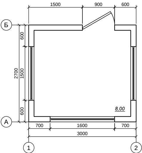
План ( 8 м²)
